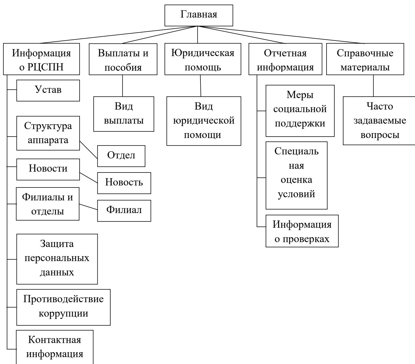
Рис. 1. Структурная схема сайта
